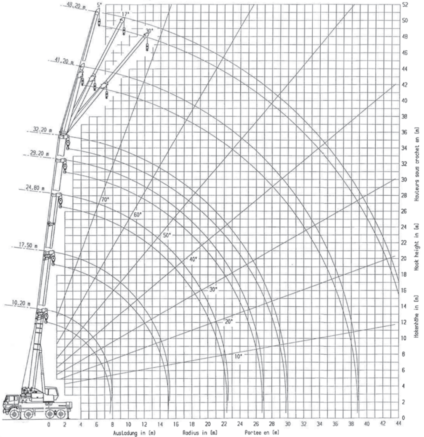
HAKENHÖHEN-KURVEN HOOK HEIGHT DIAGRAM COUBES DE HAUTEURS SOUS CROCHET
